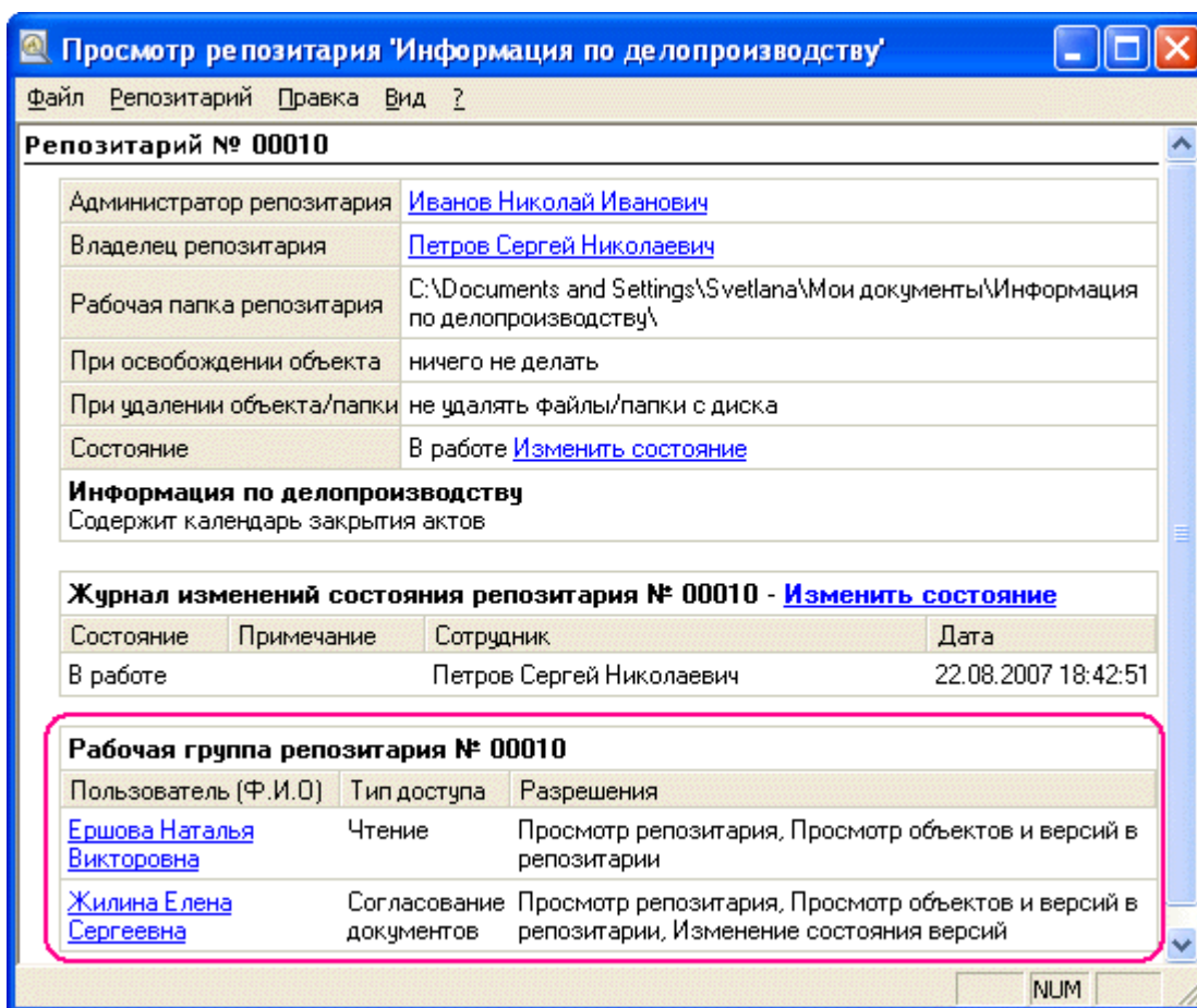
Рис.11 Просмотр рабочей группы репозитория
