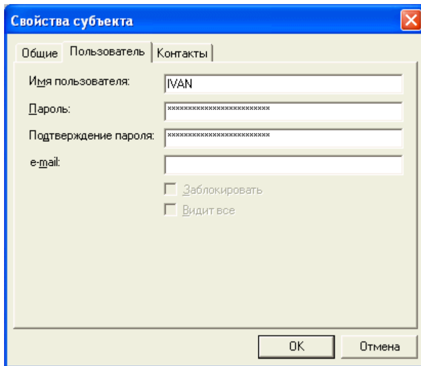
Рис.4 Свойства субъекта
