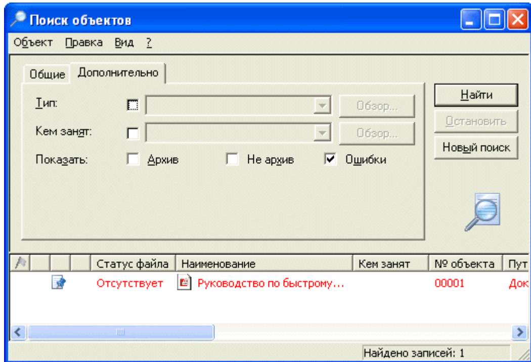
Рис.16 Форма поиска
