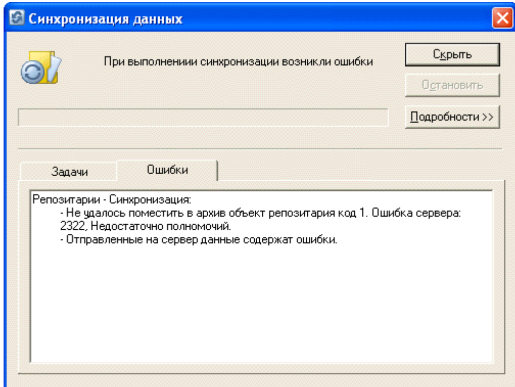
Рис.15 Диалог синхронизации
