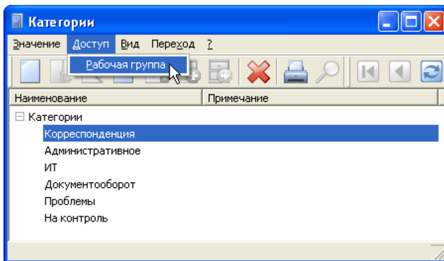
Рис.12 Справочник «Категории»
